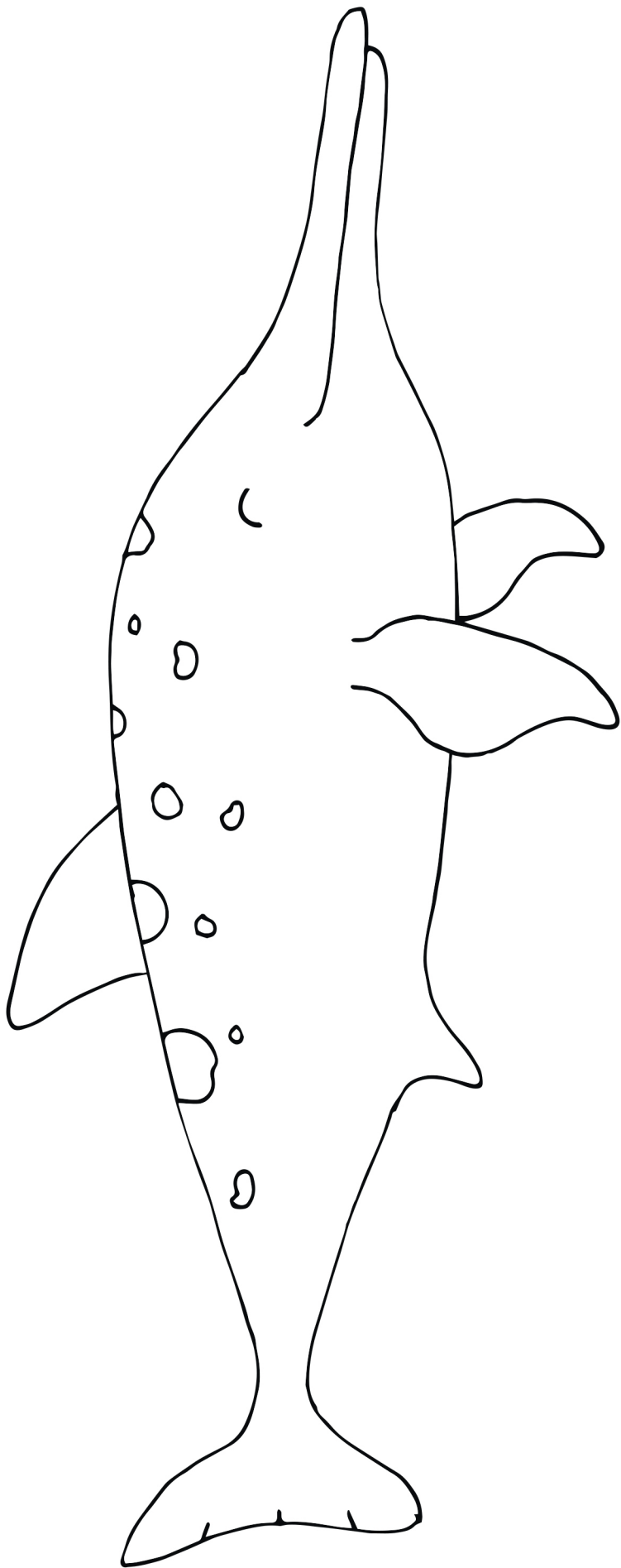
Ichthyosaurus
